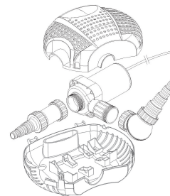
1. Filterbehuizing openen en pomp uitnemen
